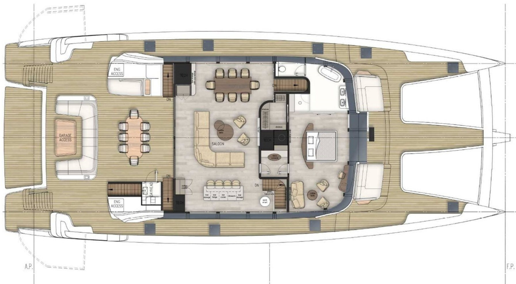
ГЛАВНАЯ ПАЛУБА
